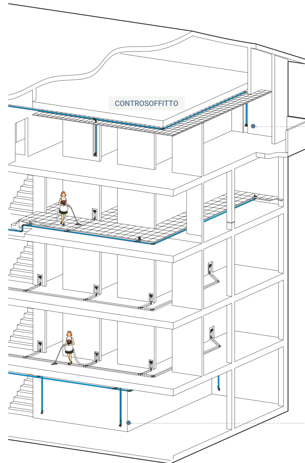
Tubazione in controsoffitto con contropresa New Air e presa New Air
